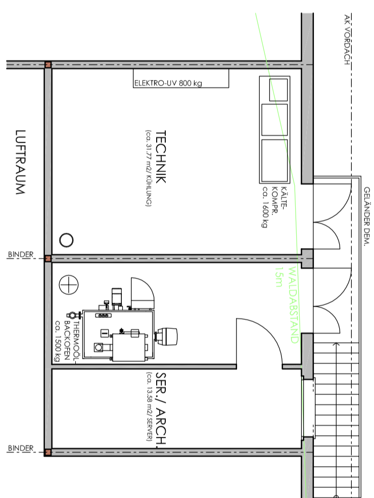
GRUNDRISS ESTRICH
